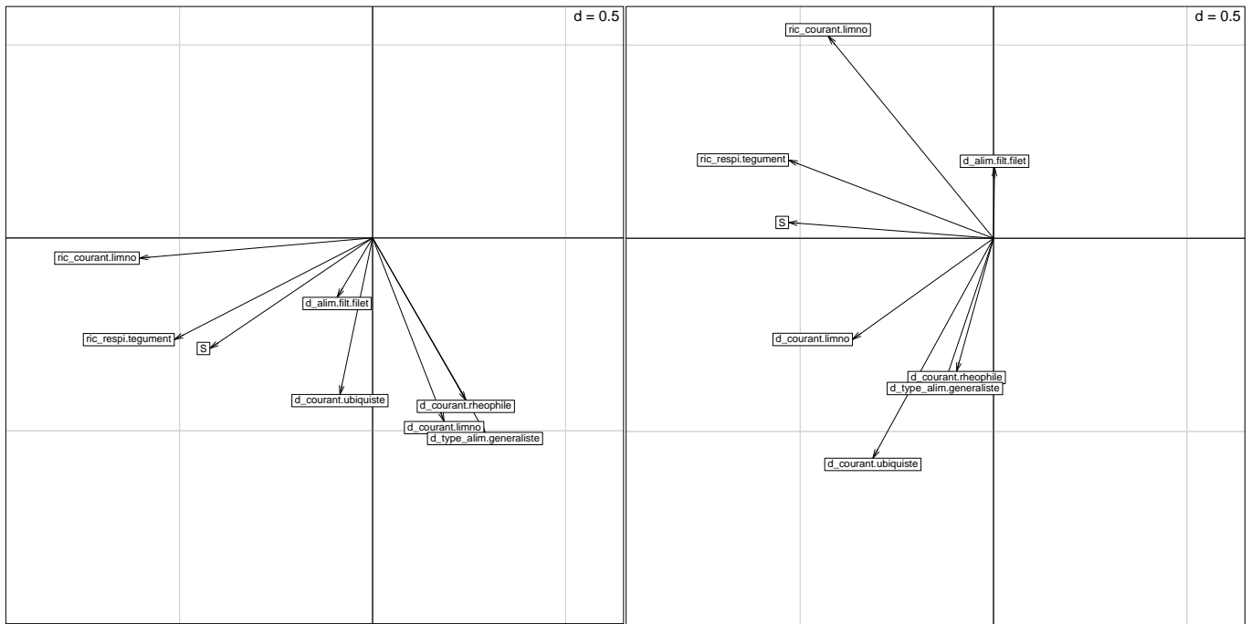
Figure 9 : Premier plan factoriel de l'ACP intra-types ref. des 8 métriques retenues. Avec : d. limnophiles : la densité en taxons limnophiles ; d. rheophiles : la densité de taxons rhéophiles ; d. ubiquiste : la densité de taxons ubiquistes d. filteurs (filet) : la densité de taxons filteurs (avec construction de filet) ; d. généralistes : la densité de taxons généralistes ; ric. limnophiles : la richesse en taxons limnophiles ; ric. tégument : la richesse en taxons à respiration tégumentaires ; S : la richesse taxonomique totale. A gauche sans la transformation logarithmique, à droite avec la transformation logarithmique.
