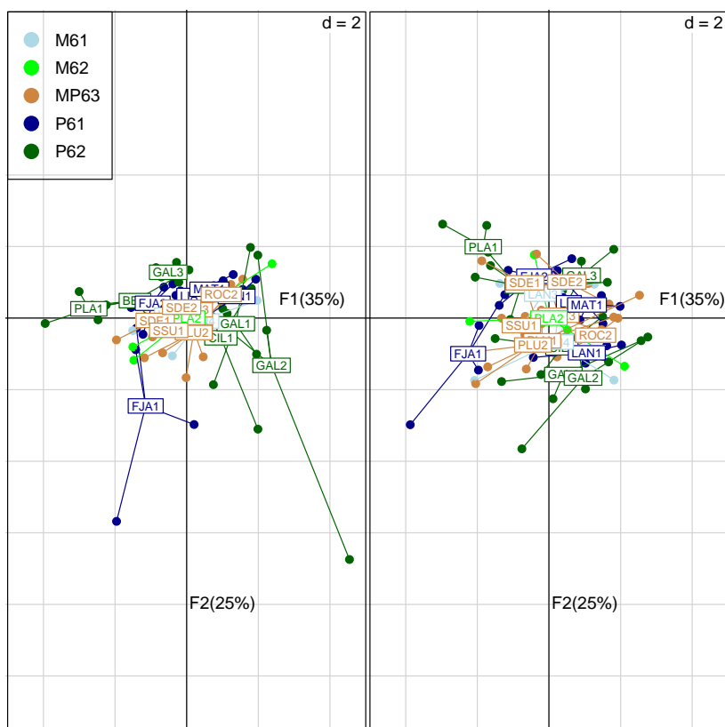
Figure 8 : Premier plan factoriel de l'ACP intra-types ref. Chaque point correspond à une station-campagne « référence » à partir du référentiel 2. Chaque station est positionnée au barycentre des stations-campagnes. Les couleurs regroupent les stations selon leur type de masses d'eau. A gauche sans la transformation logarithmique, à droite avec la transformation logarithmique.
