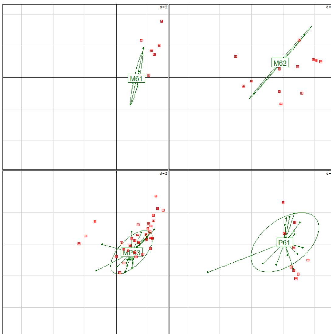
Figure 6 : Projection en individus supplémentaires des stations-campagnes « test » (carrés rouges) sur le premier plan factoriel de l'ACP ref. La distribution des valeurs de référence est représentée par une ellipse illustrant la variabilité au sein de chaque type. Les deux types P62 et MP64 ne sont pas représentés (pas de station « test » ou de référence, Tableau 6).
